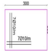
لوح من خزان الصرف
