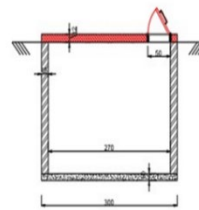
قسم من خزان الصرف الصحي
